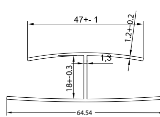
H PROFIL
